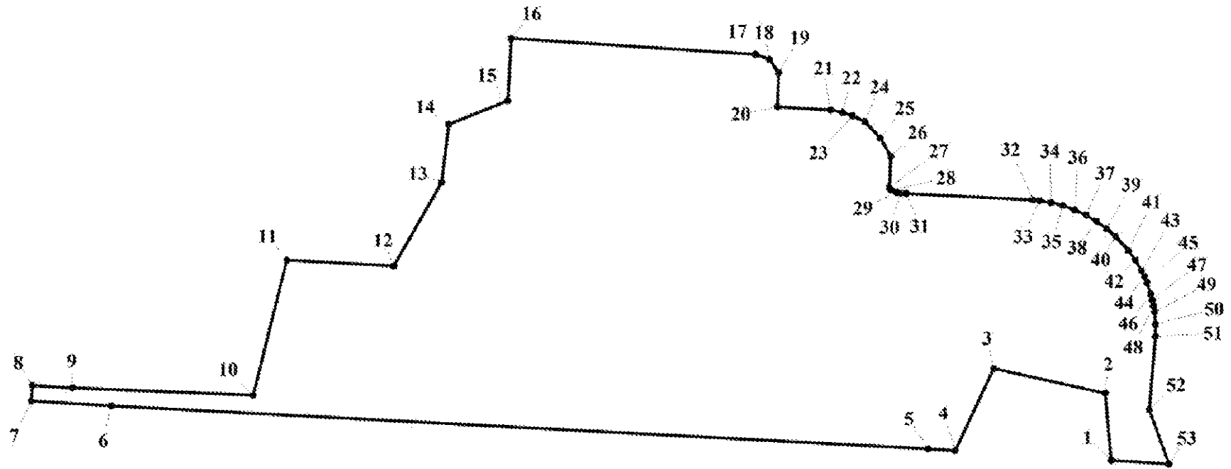
Разбивочный план границ образуемого земельного участка
